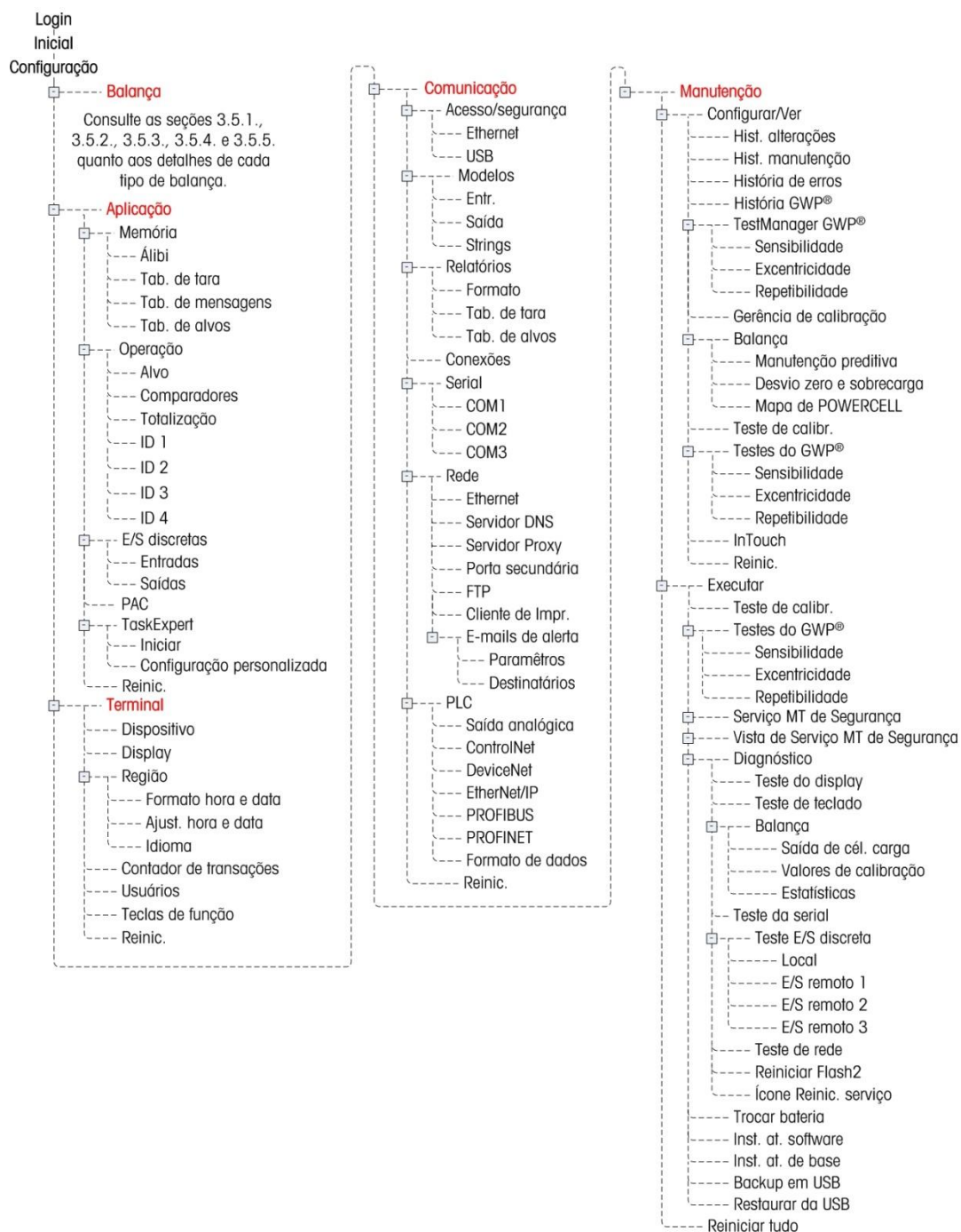
Figura 3-5: A Árvore do Menu do IND570 com Todos os Ramos Possíveis Expandidos
