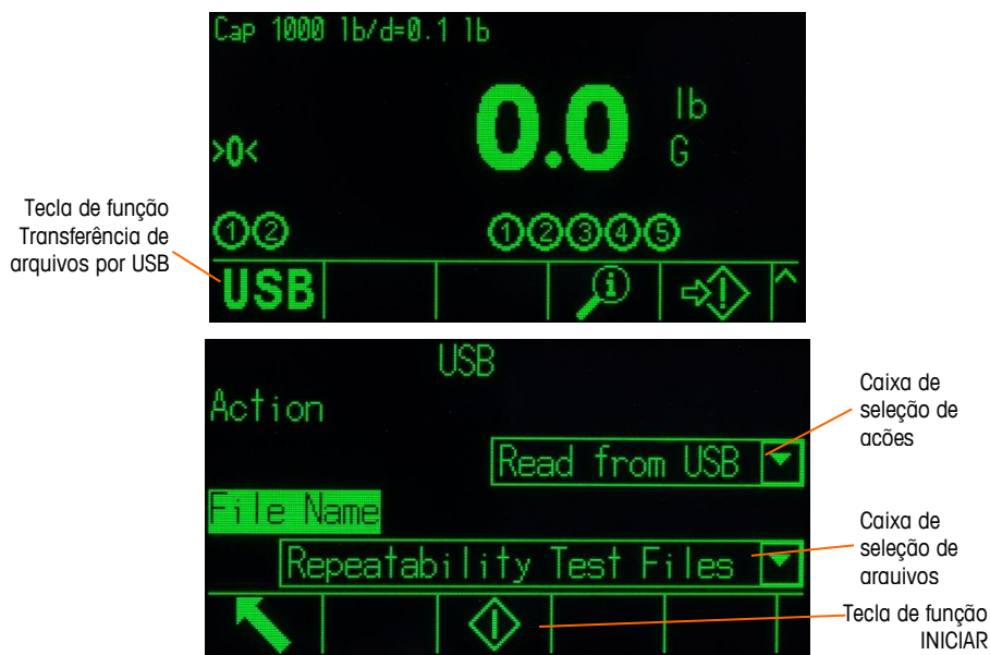
Figura 2-32: Telas de Função de Transferência de Arquivo por USB e Seleção de Arquivos
