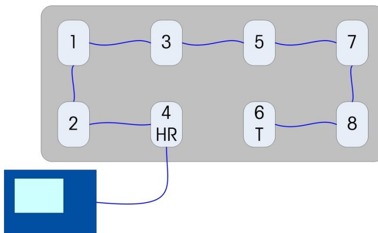
Figura 3-25: Esquema da Rede POWERCELL
