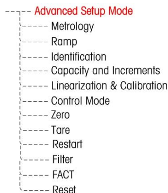
Figura 3-8: Estrutura básica do modo de configuração avançada
