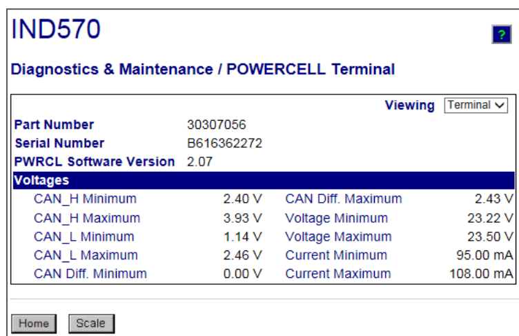
Figura 5-30: Dados de Terminal POWERCELL
