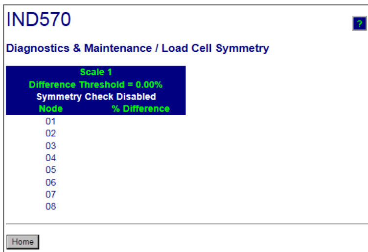
Figura 5-29: Simetria de Célula de Carga
