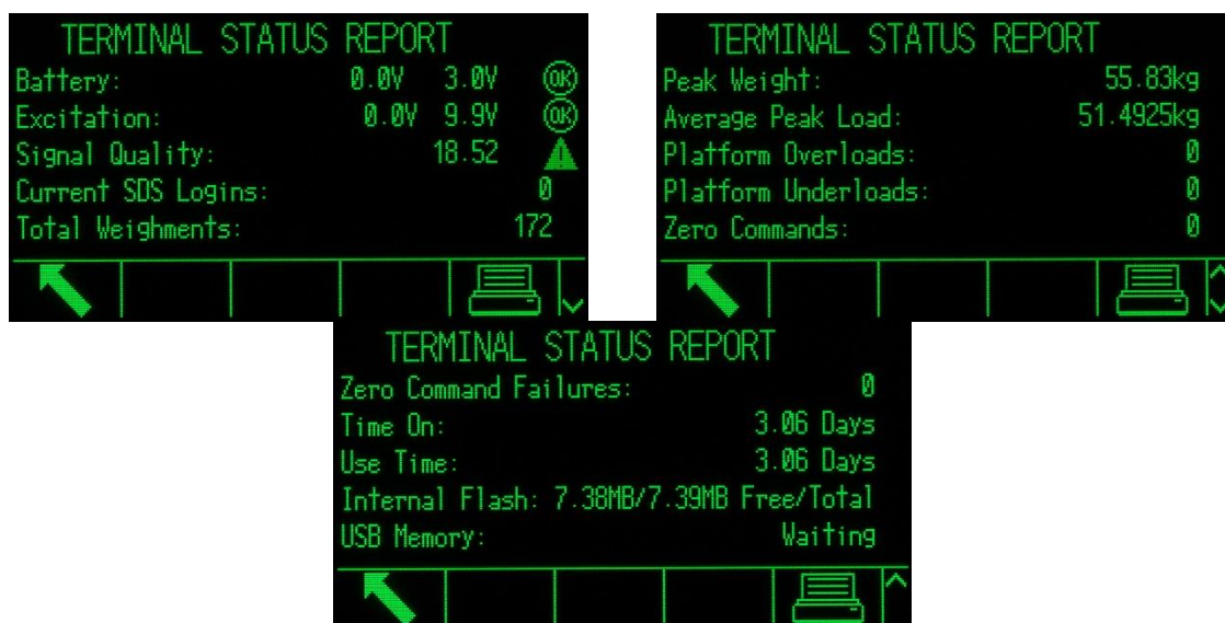
Figura 4-10: Relatório de Status do Terminal
