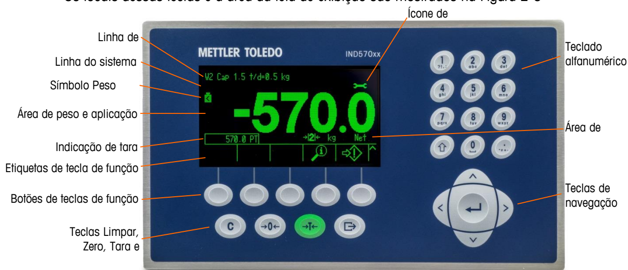
Figura 2-5: Localizações de teclas e tela de exibição
