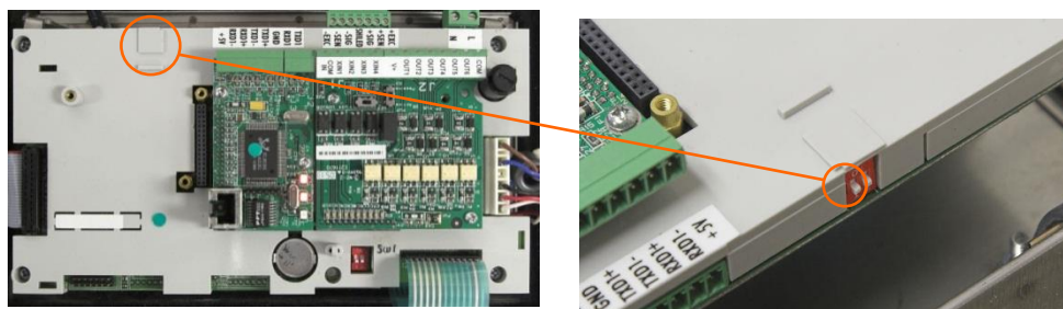
Figura 5-33: Localização da Chave SW2-1
