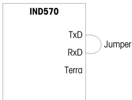
Figura 5-10: Fio de Jumper entre os Terminais de Transmissão e Recepção
