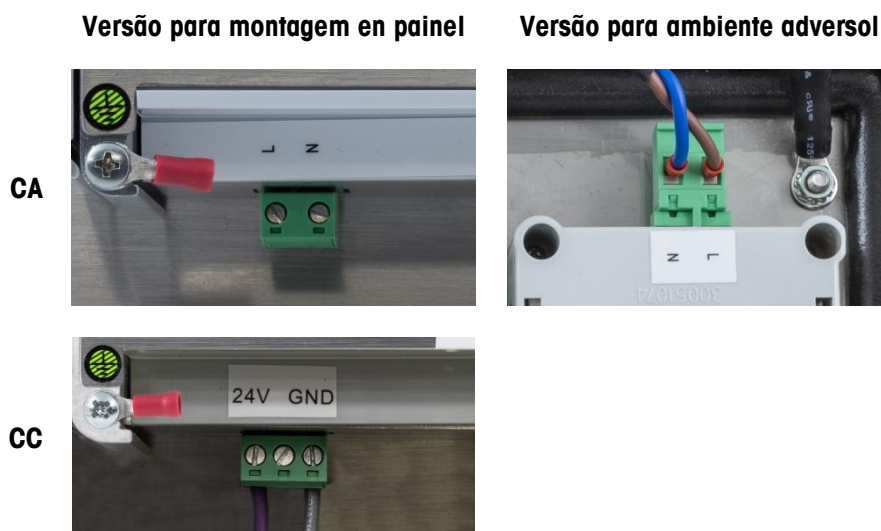
Figura 5-8: Pontos de Teste de Alimentação CA e CC - Painel (esquerda) e Para ambiente adversol (direita)
