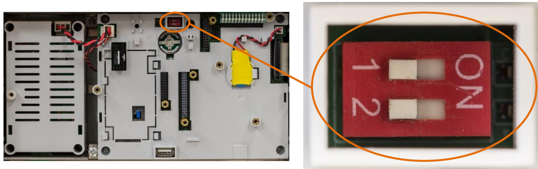
Figura 2-4: Localização da Chave de Metrologia
