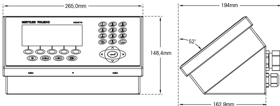
Figura 1-5: Dimensões do Gabinete para Ambiente Adverso, IND570
