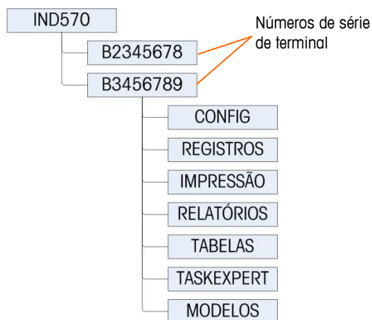
Figura 2-33: Estrutura de Arquivos USB
