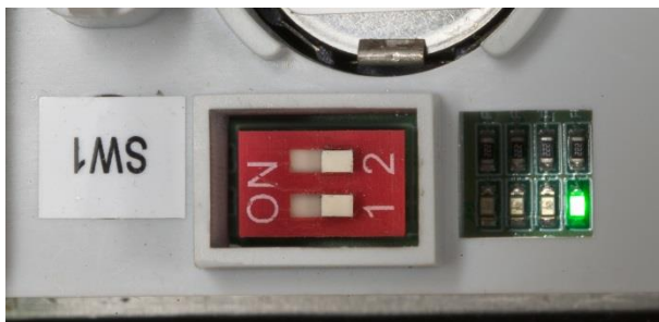
Figura 5-5: Posição de LED 4 na Placa de Circuito Impresso Principal
