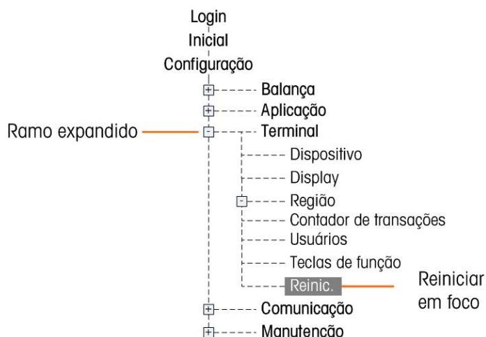
Figura 3-29: Árvore do Menu de Configuração - Reiniciar
