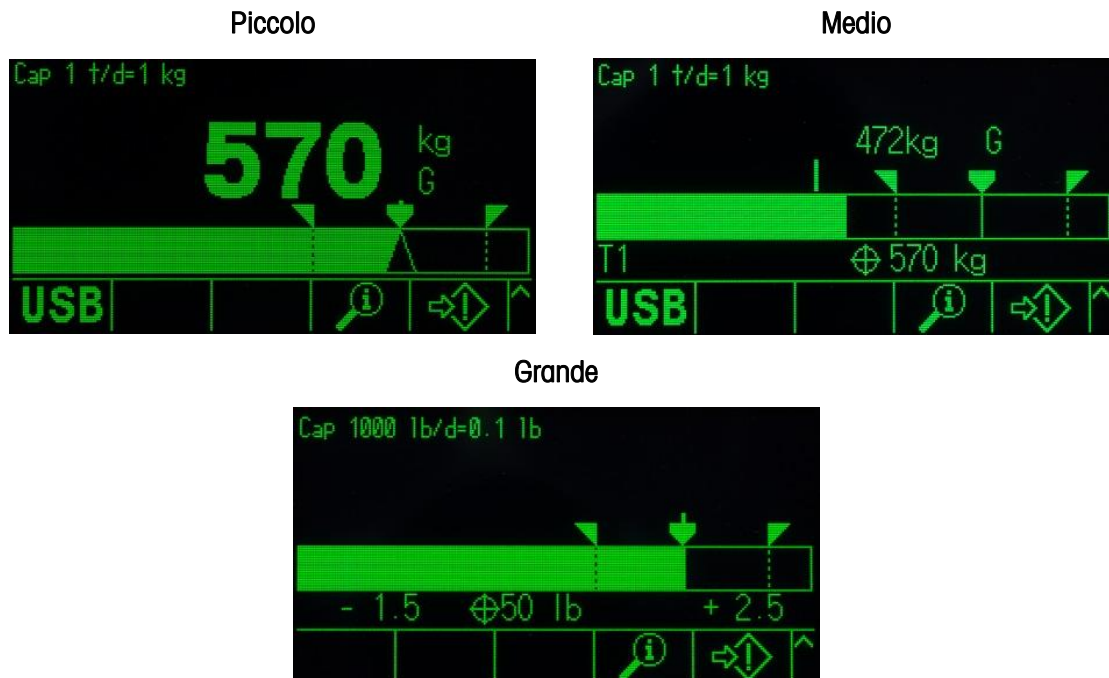
Figura 4-17: Dimensioni del Display SmartTrac in Trasferimento materiale
