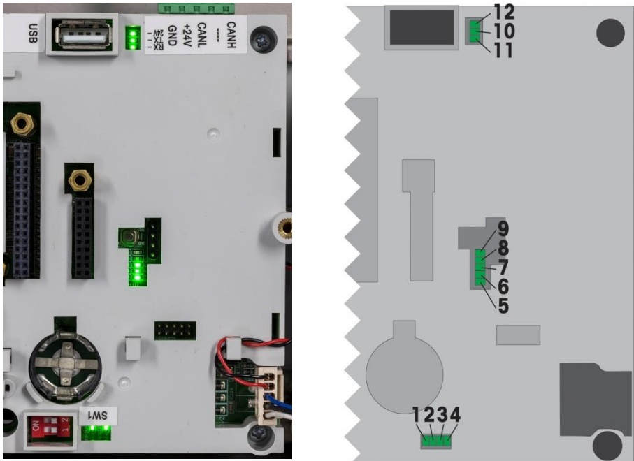
Figura 5-6: LED scheda principale POWERCELL
