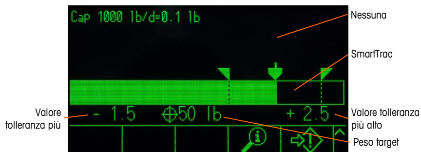
Figura 2-22: Trasferimento materiale SmartTrac, Grande
