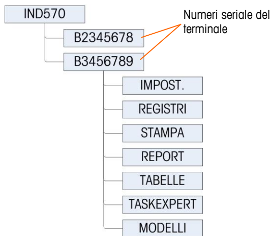
Figura 5-1: Struttura dei file del backup su USB
