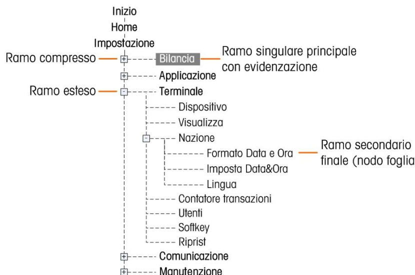
Figura 3-2: Esempio di struttura del menu di impostazione
