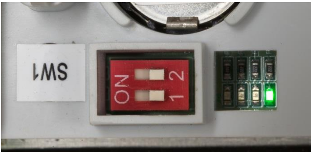
Figura 5-5: Posizione del LED 4 sul PCB della scheda principale
