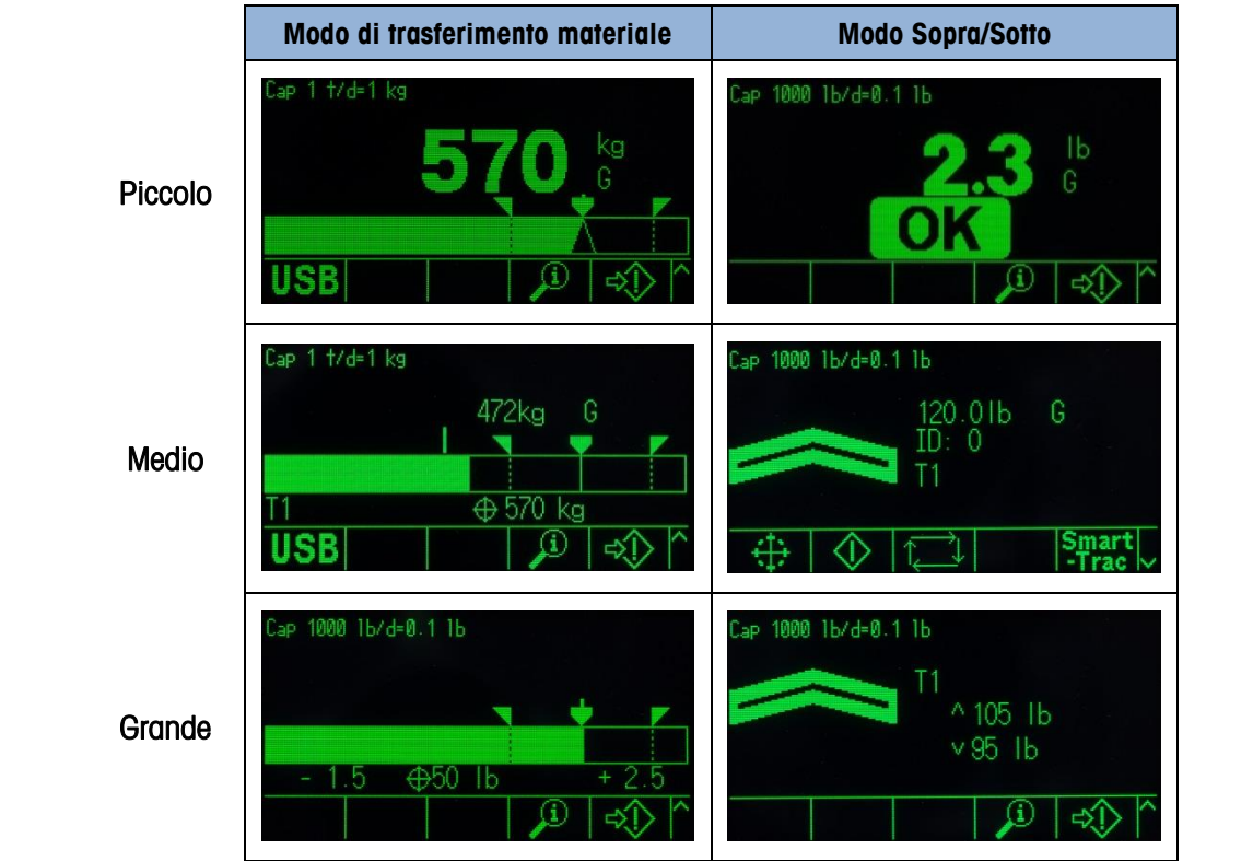
Figura 3-14: Dimensioni del Display SmartTrac, Trasferimento materiale e Sopra/Sotto
