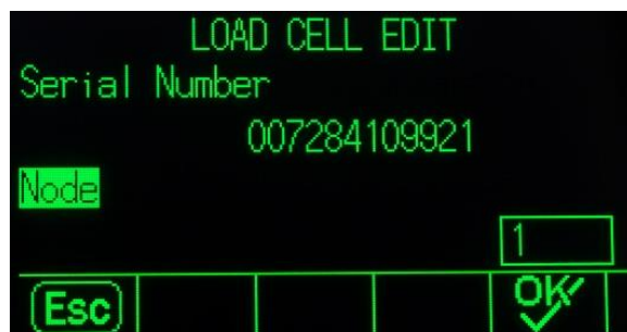
Figura 3-11: schermata di modifica dell'assegnazione dell'indirizzo manuale delle celle di carico
