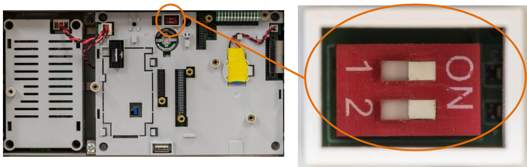
Figura 5-32: Posizione dell'interruttore metrologia
