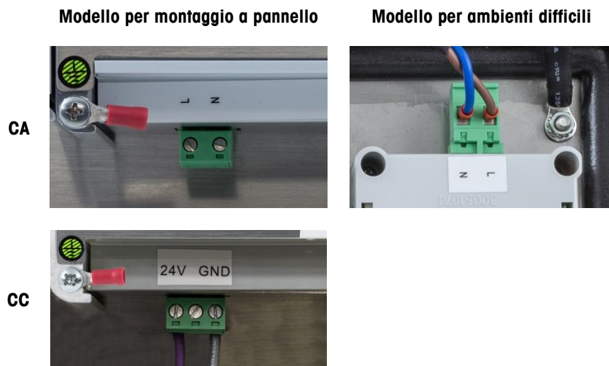
Figura 5-8: Punto di prova dell'alimentazione in CA – Pannello (sinistra) e ambienti difficili (destra)
