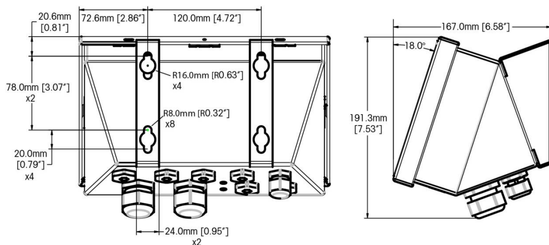
Figura 1-7: Dimensioni dell'armadietto per ambienti difficili IND570, con staffe di montaggio ad angolo fisso – montaggio originale
