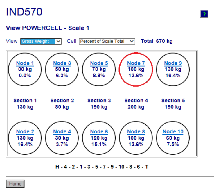
Figura 5-26: Pagina sui dati e la mappa della bilancia POWERCELL
