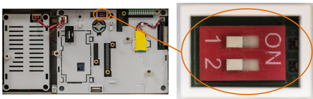
Figura 2-4: Posizione dell'interruttore Metrologia
