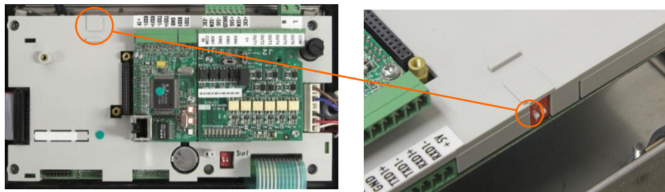
Figura 5-33: Posizione dell'interruttore SW2-1
