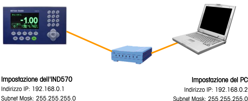
Figura C-1: Esempio di configurazione Indirizzo IP
