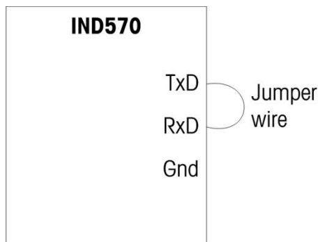
Figura 5-10: Ponticello tra i terminali di trasmissione e ricezione
