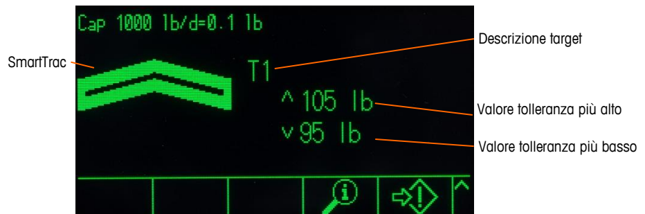
Figura 2-26: Display Sopra/Sotto, grande
