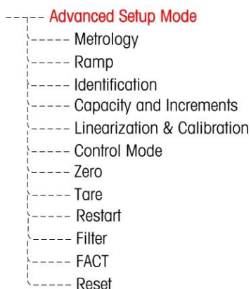
Figura 3-8: Struttura del menu di base, modalità di impostazione avanzata
