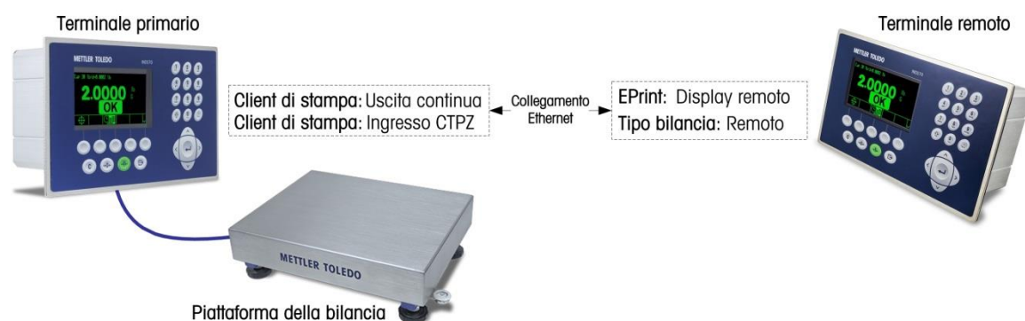
Figura 4-16: Esempio di configurazione del terminale per la funzione di display remoto tramite Ethernet
