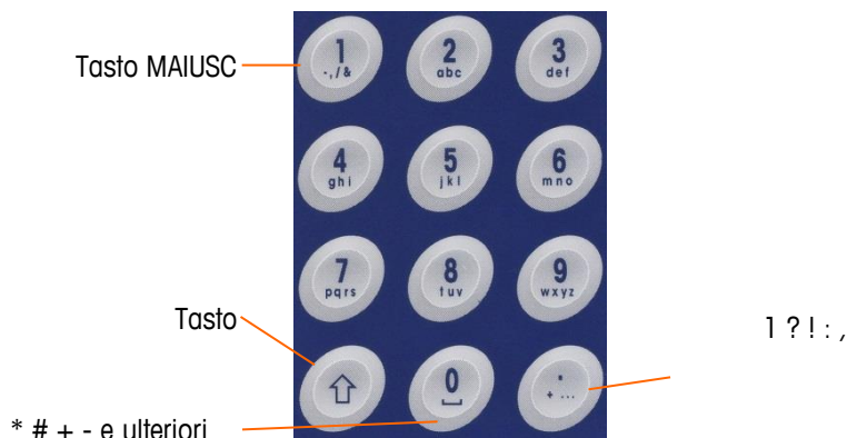
Figura 2-7: Struttura tastierino alfanumerico
