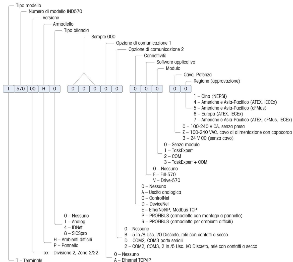
Figura 1-1: Identificazione SCK IND570
