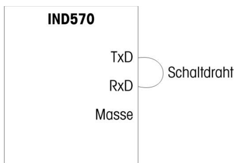
Abbildung 5-10: Drahtbrücke zwischen der Sende- und Empfangsklemme
