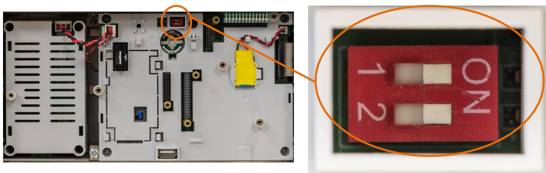
Abbildung 5-32: Position des Metrologieschalters
