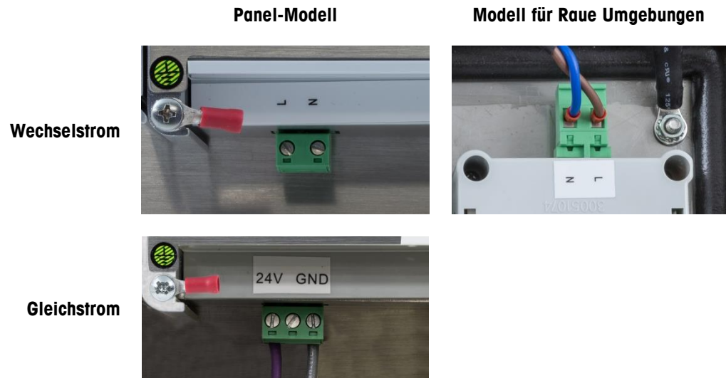
Abbildung 5-8: Netzspannungs-Prüfpunkt - Frontplattenausführung (links) und Ausführung für raue Umgebungen (rechts)
