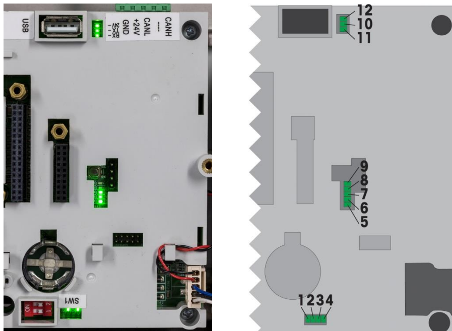
Abbildung 5-6: LEDs auf der POWERCELL-Hauptplatine
