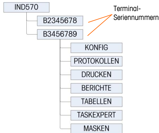
Abbildung 2-33: USB-Dateistruktur
