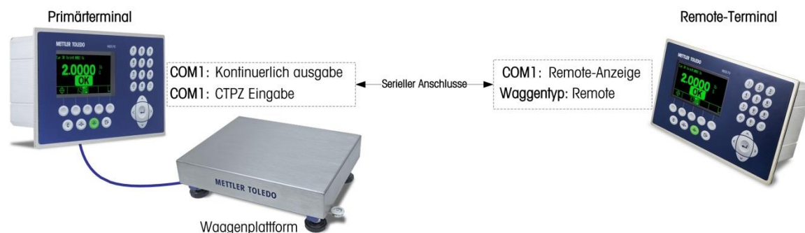
Abbildung 2-16: Fernanzeigefunktion über serielle Schnittstelle
