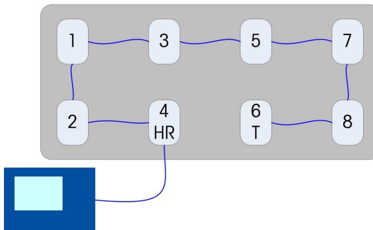
Abbildung 3-25: Skizze des POWERCELL-Netzwerkes
