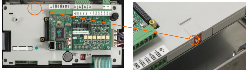
Abbildung 5-33: Position des Schalters SW2-1
