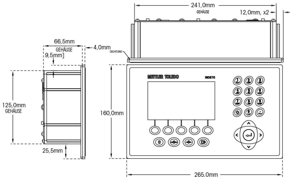
Abbildung 1-3: Gehäuseabmessungen der IND570-Frontplattenversion
