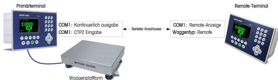
Abbildung 4-15: Beispiel für die Terminalkonfiguration mit Fernanzeige über serielle Verbindung
