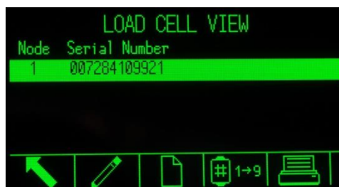
Abbildung 3-10: Bildschirm mit Ansicht der manuellen Adressierung der Wägezellen
